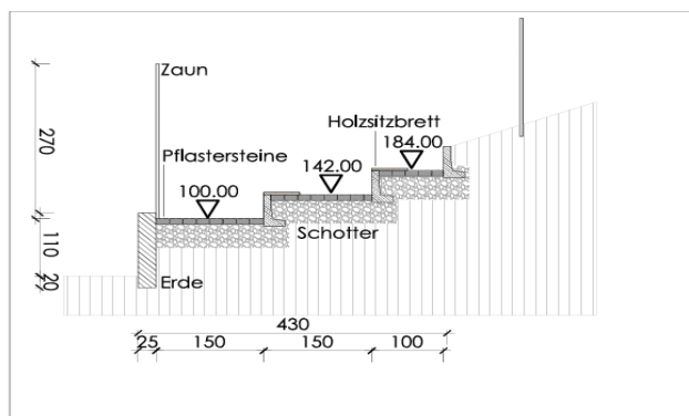
Schnitt 1.50
